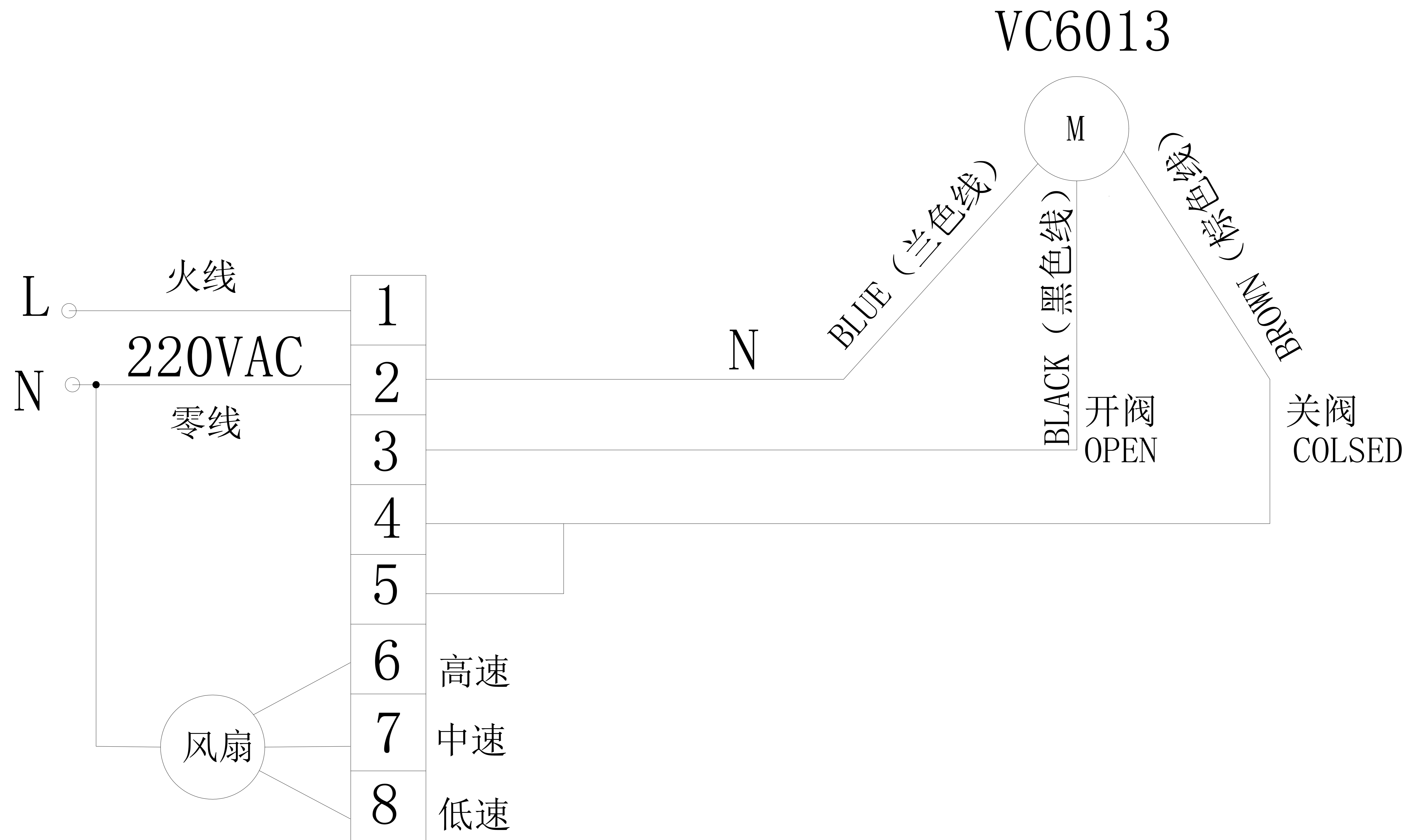
T6373B接线端子
